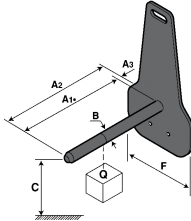
EPE: Auslegearm
