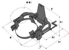
FUT: Fasswender
