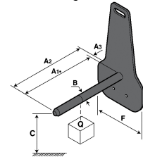
EPE: Auslegearm
